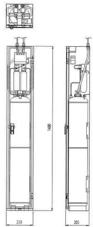
CPW13161
